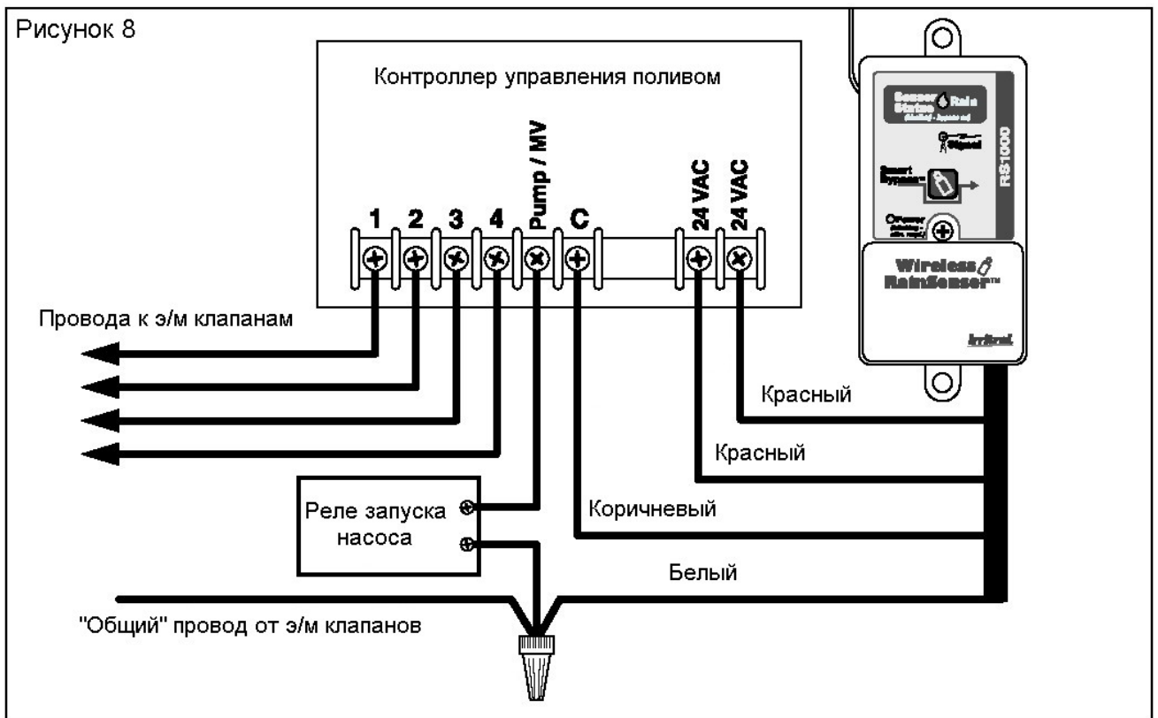
Рисунок 8 : Схема присоединения к контроллеру, в котором нет специальных разъемов для подключения датчика дождя. В системе полива также используется «Реле запуска насоса» или «мастер-клапан».
